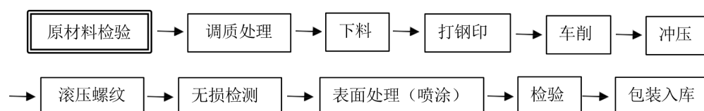
图 1 风电机组叶片用高强度螺柱生产工艺流程图
