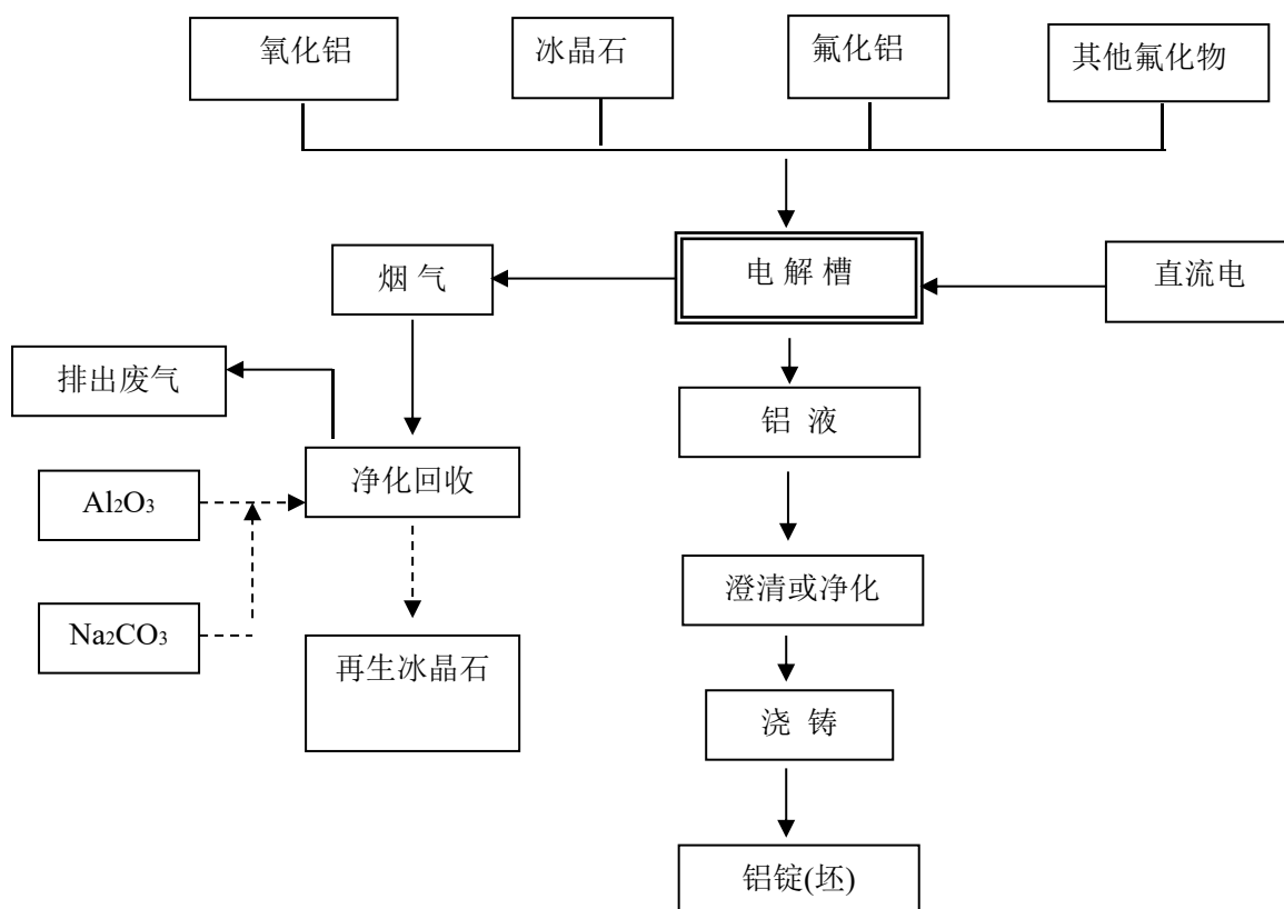
图1 重熔用铝锭生产工艺流程图
